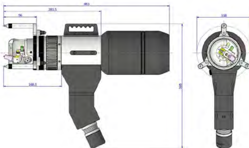
Dimensionen TSH 16
